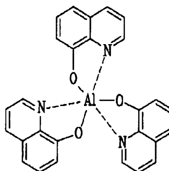
Alq3
