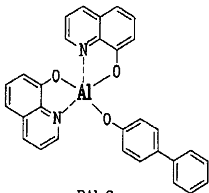
BAlq3
